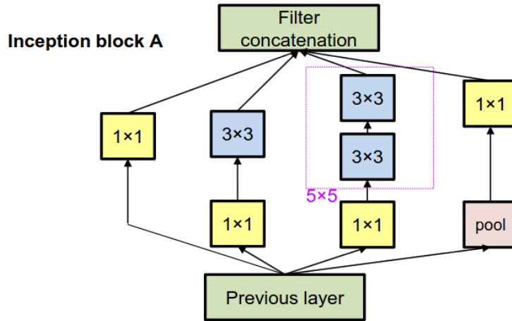
Figura 8: Bloco Inception v2 A
