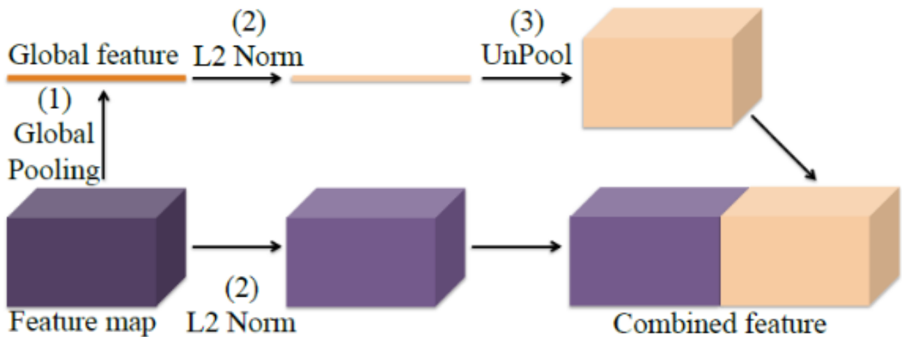
Figura 23: Exemplo de image pooling
