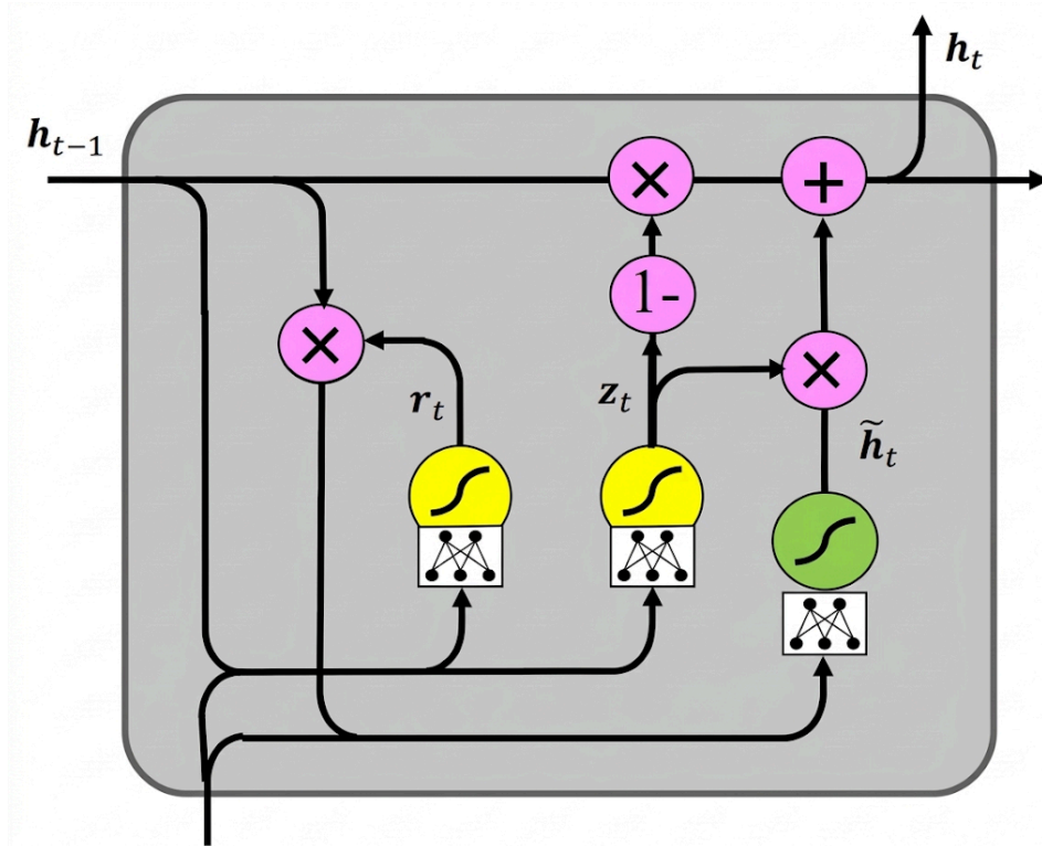
Figura 64: Arquitetura de uma célula GRU
