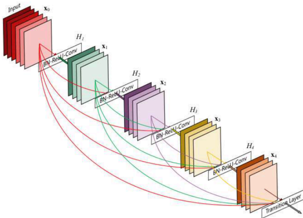
Figura 12: Arquitetura da DenseNet
