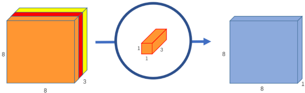
Figura 28: Exemplo de pointwise convolution com 3 canais
