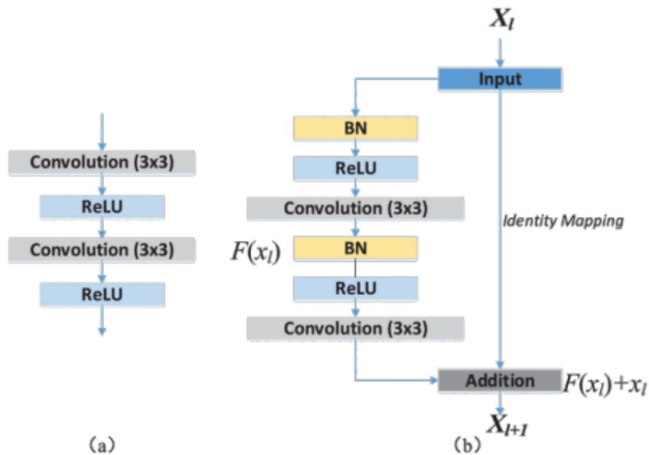
Figura 33: (a) Bloco padrão da UNet. (b) Bloco residual da ResUNet
