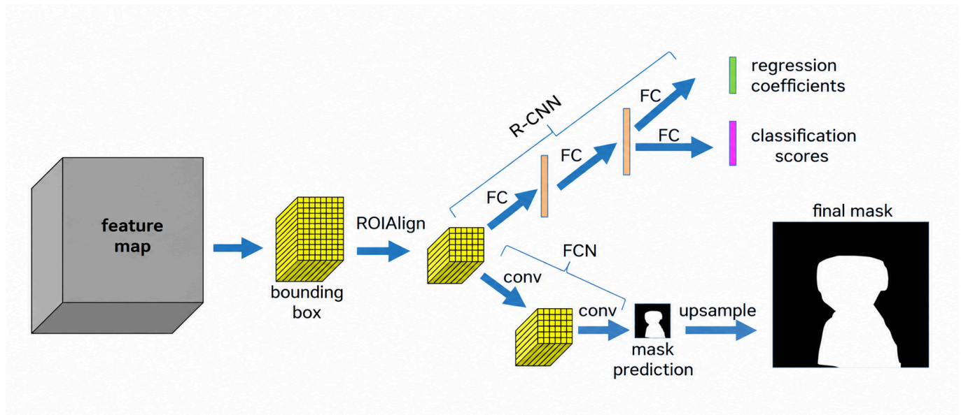
Figura 49: Arquitetura da Mask R-CNN com predições em paralelo
