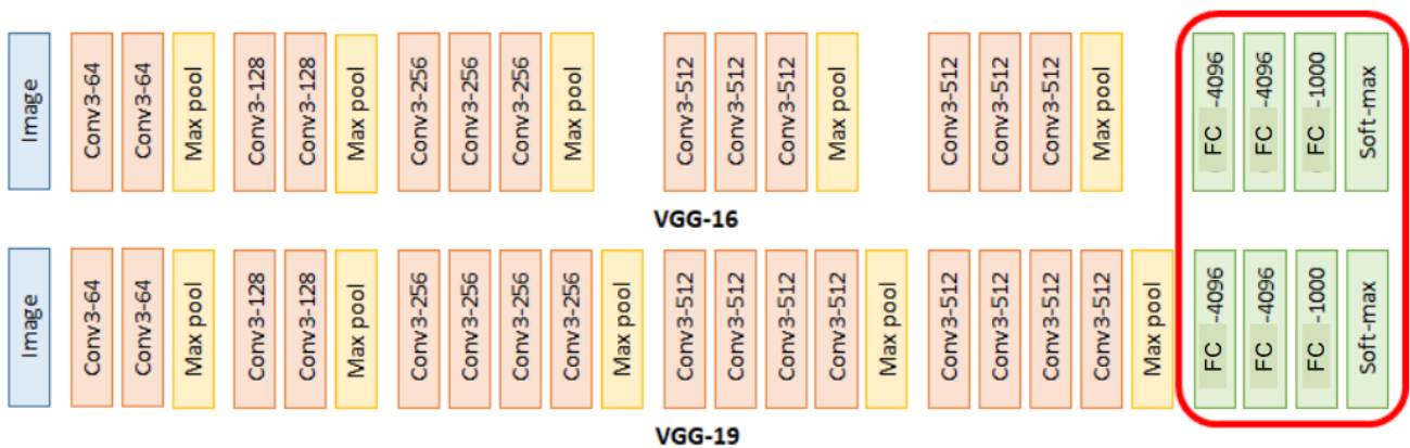
Figura 5: Arquitetura da VGGNet
