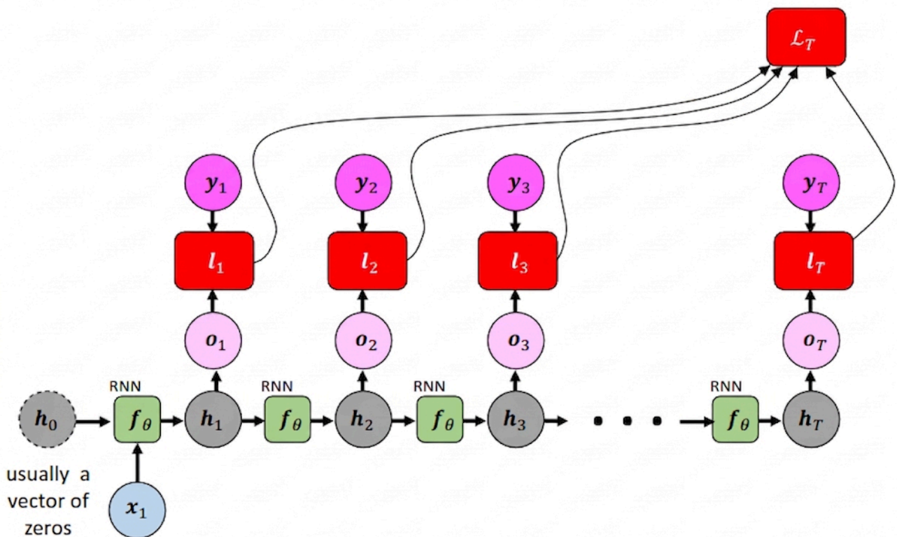
Figura 58: Exemplo de mapeamento one-to-many
