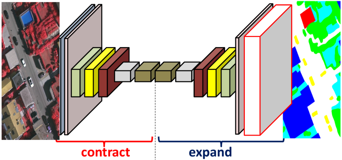
Figura 19: Estrutura de uma rede encoder-decoder
