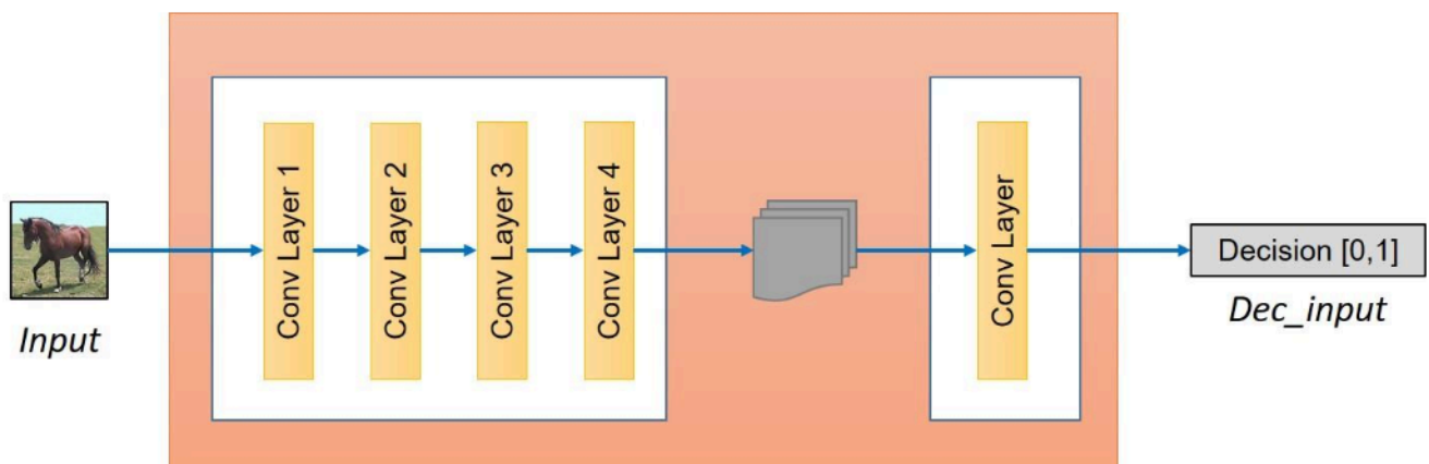
Figura 77: Arquitetura dos discriminadores em CycleGANs
