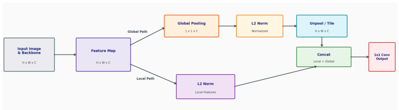
Figura 35: Arquitetura simplificada da PARSENet
