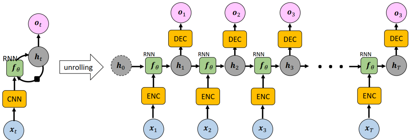
Figura 65: Arquitetura de uma CNN seguida por uma RNN
