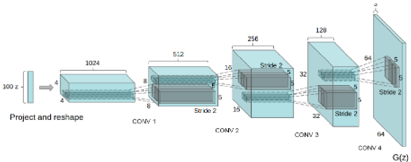
Figura 69: Arquitetura de uma DCGAN
