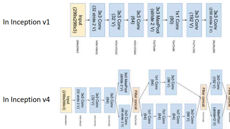
Figura 10: Arquitetura da Inception v4
