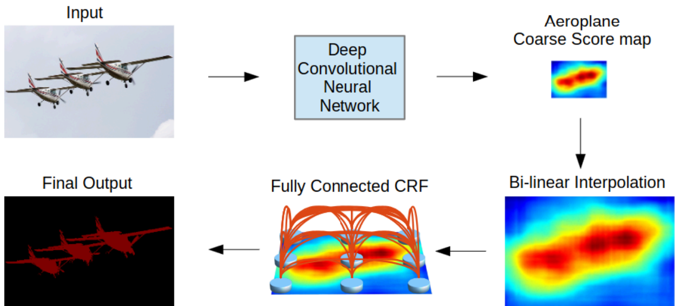
Figura 34: Arquitetura da DeepLabV1&V2
