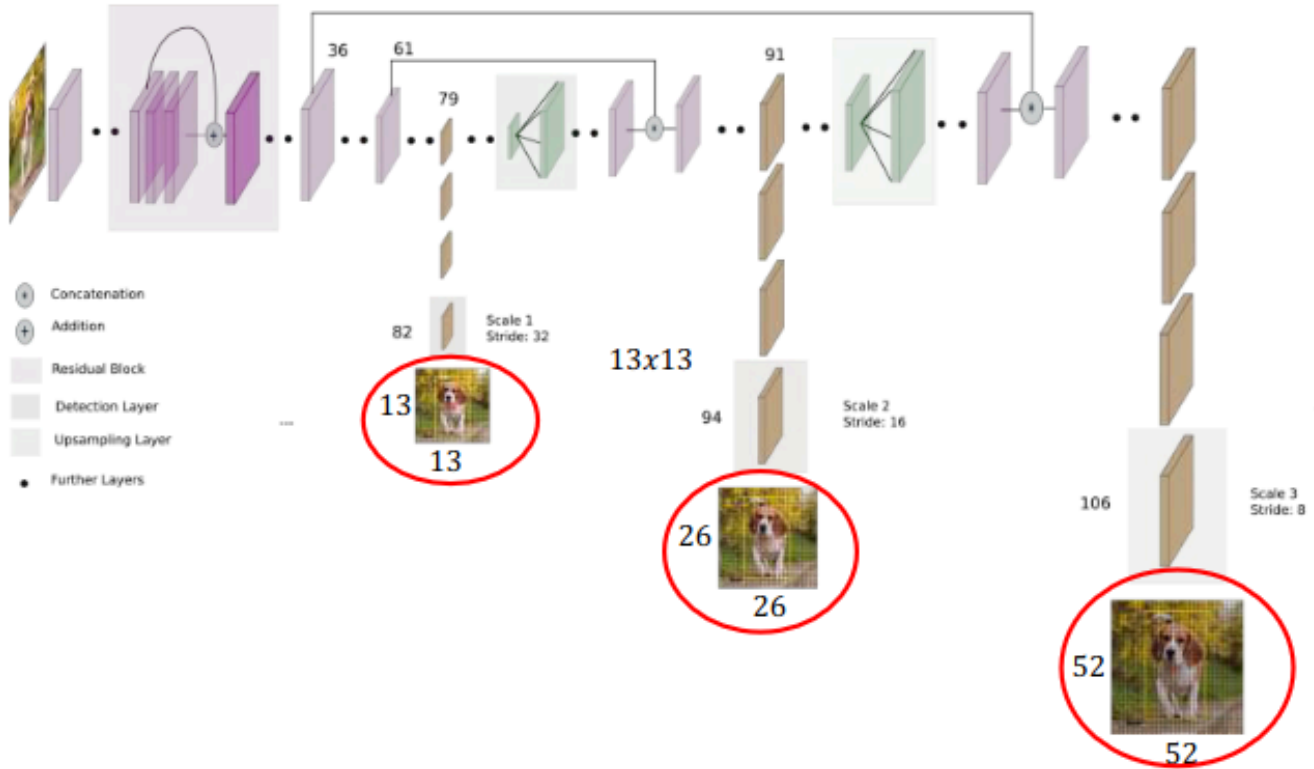
Figura 44: Arquitetura da YOLOv3
