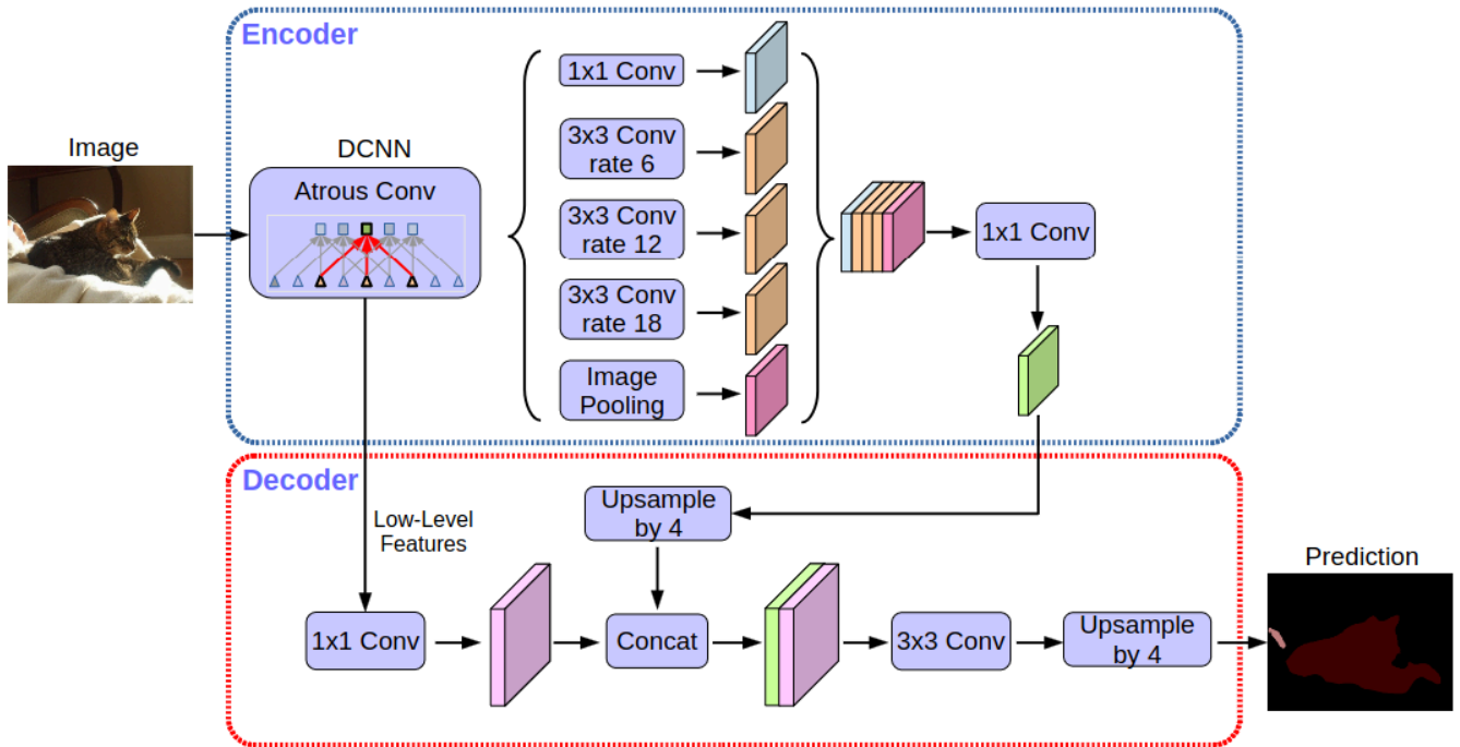
Figura 38: Arquitetura da DeepLabV3+
