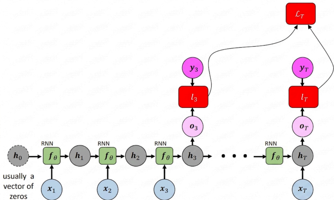
Figura 57: Exemplo de mapeamento many-to-many
