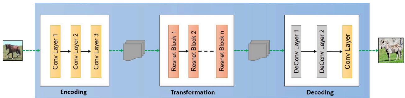
Figura 75: Arquitetura dos geradores em CycleGANs
