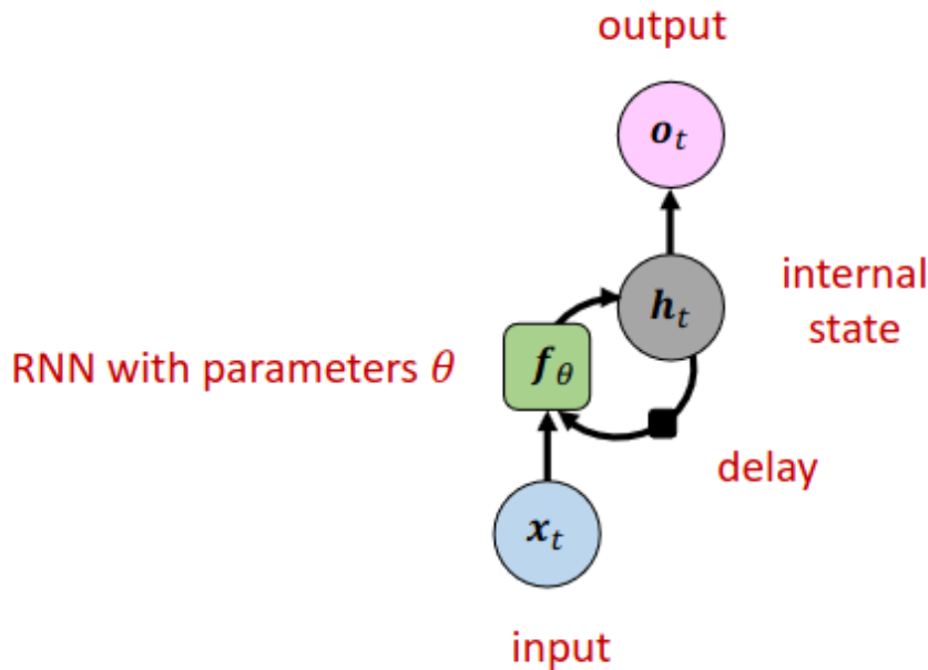
Figura 54: Arquitetura de uma RNN
