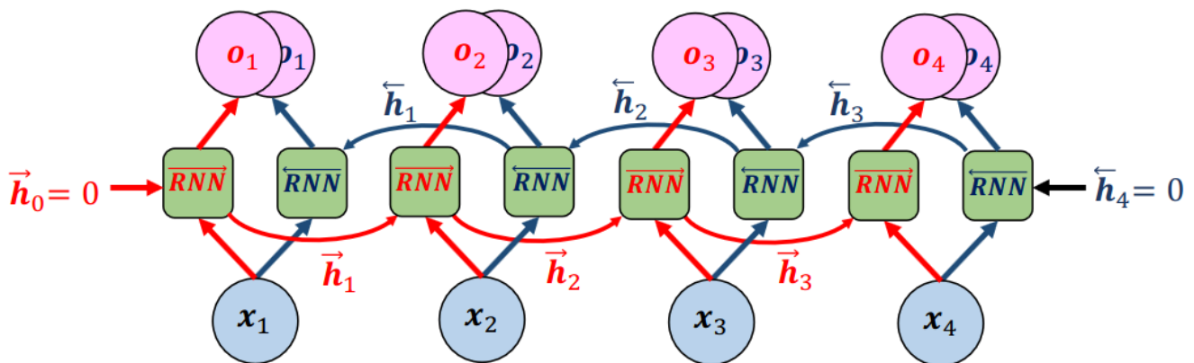
Figura 66: Arquitetura de uma RNN Bidirecional
