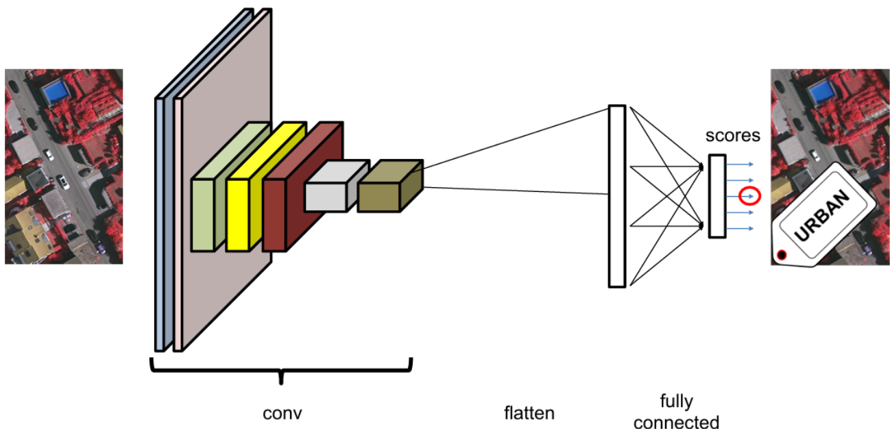
Figura 16: Estrutura de uma rede convolucional padrão
