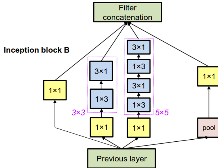
Figura 9: Bloco Inception v2 B
