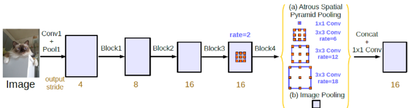
Figura 37: Arquitetura da DeepLabV3
