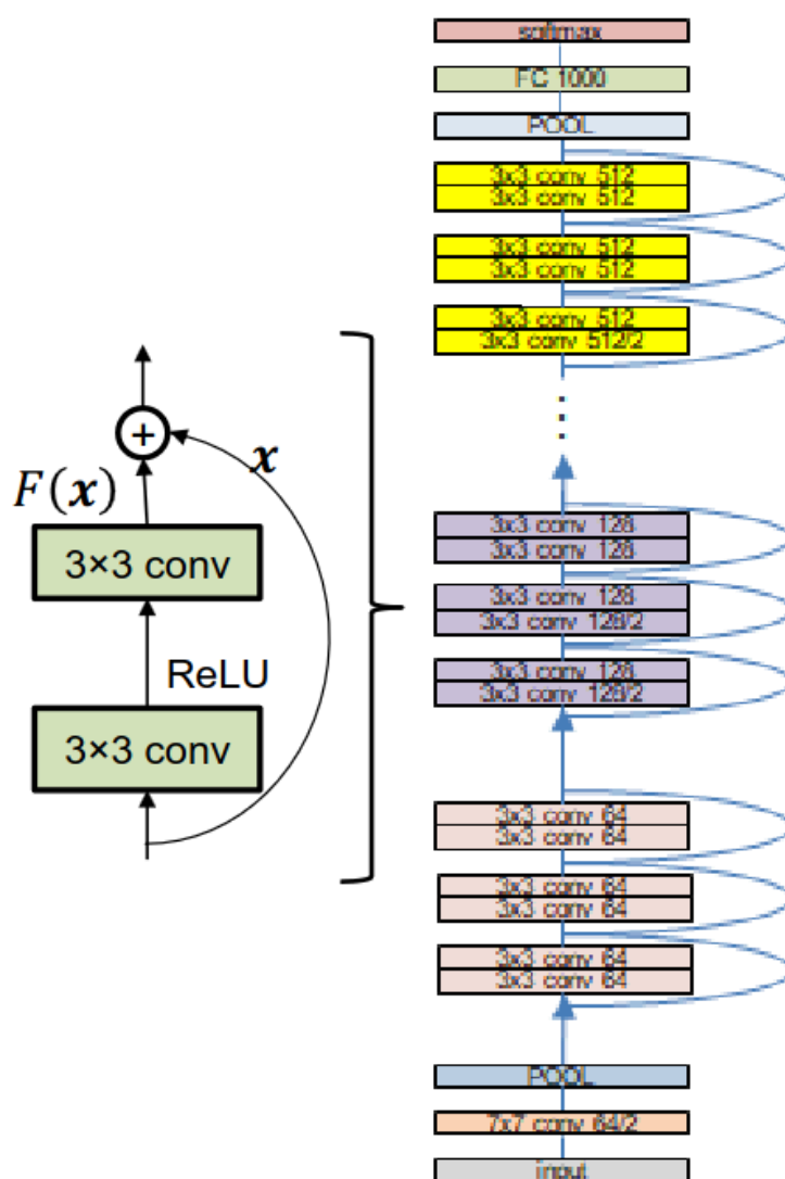
Figura 11: Arquitetura da ResNet
