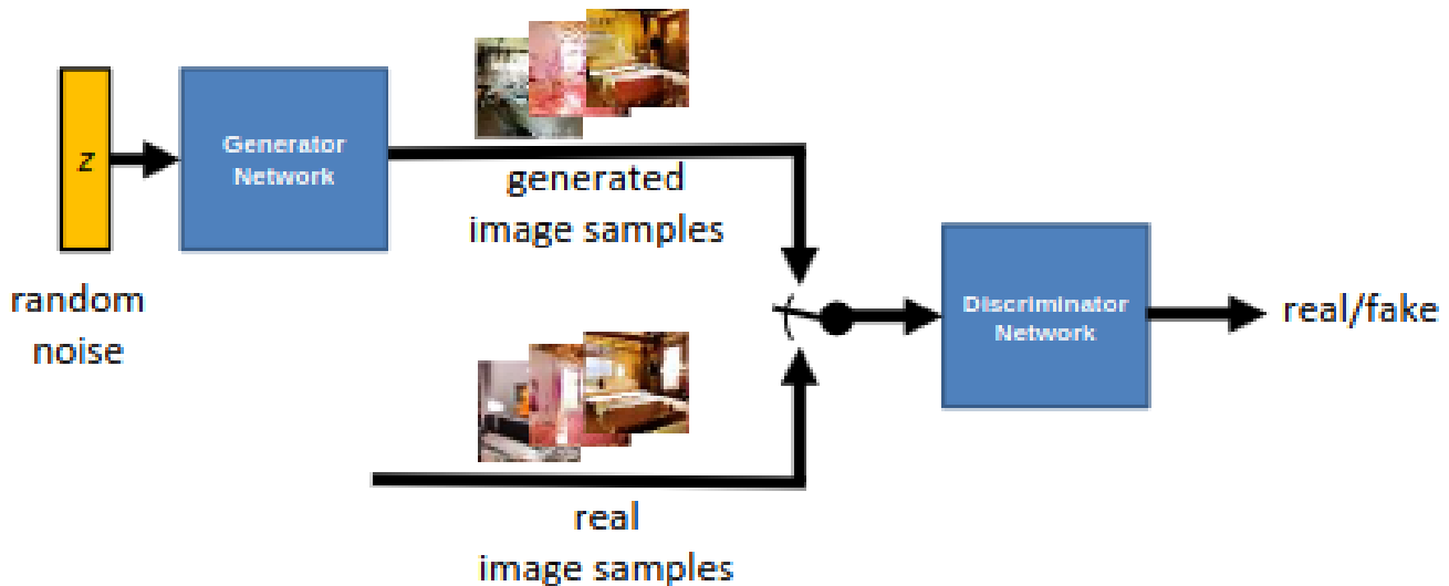
Figura 68: Arquitetura de uma GAN
