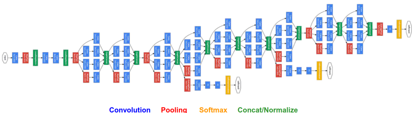
Figura 6: Arquitetura da GoogLeNet (Inception v1)
