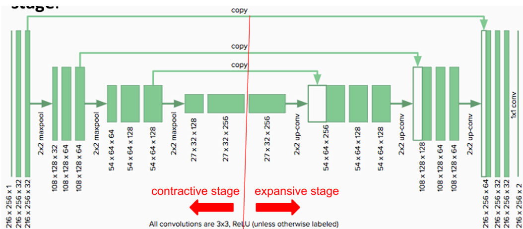
Figura 31: Arquitetura da U-Net
