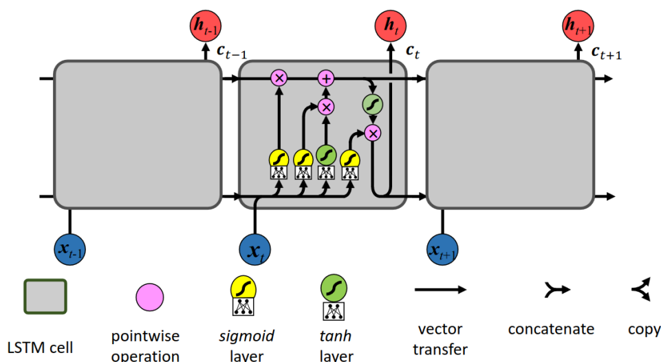
Figura 63: Arquitetura de uma célula LSTM
