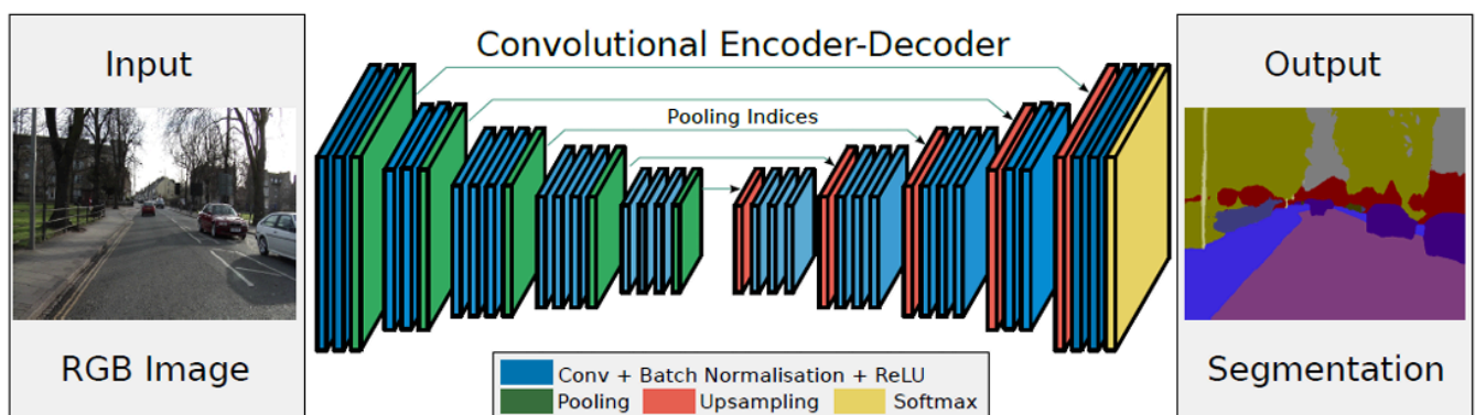
Figura 30: Arquitetura da SegNet
