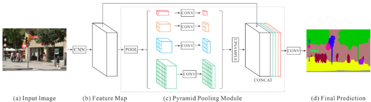
Figura 36: Arquitetura da PSPNet
