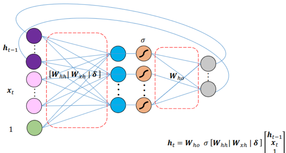
Figura 53: Bloco de uma RNN
