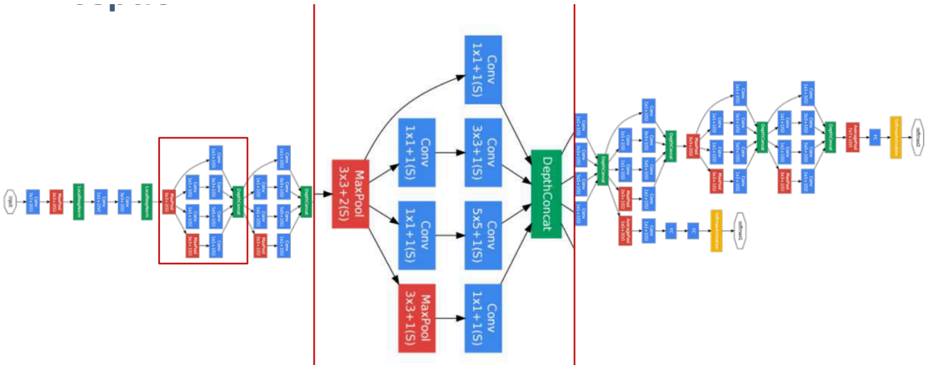
Figura 7: Módulo Inception da GoogLeNet
