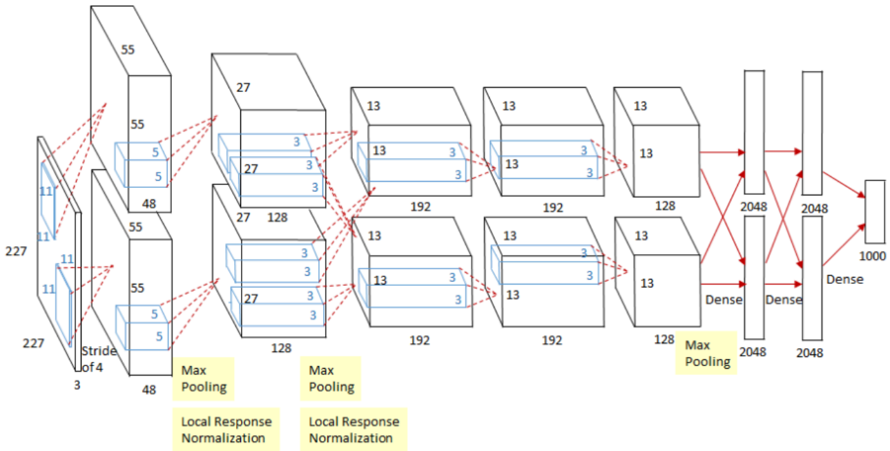
Figura 4: Arquitetura da AlexNet
