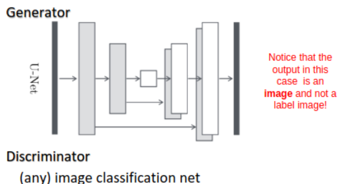
Figura 71: Arquitetura de uma cGAN clássica (pix2pix)
